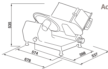
Dimensions Gravinox 350
