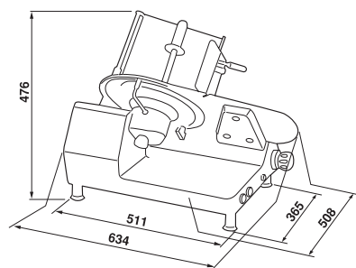
Dimensions Gravinox 300
